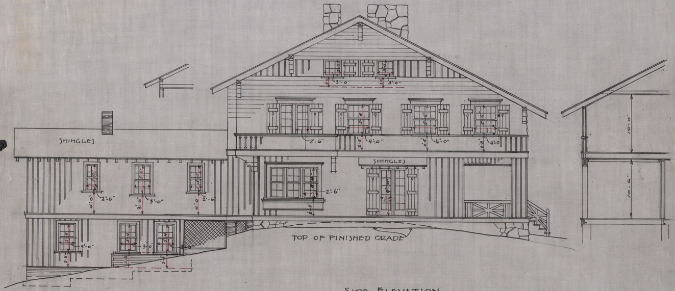
SIDE ELEVATION SCALE: 1/8"=1'-0"
